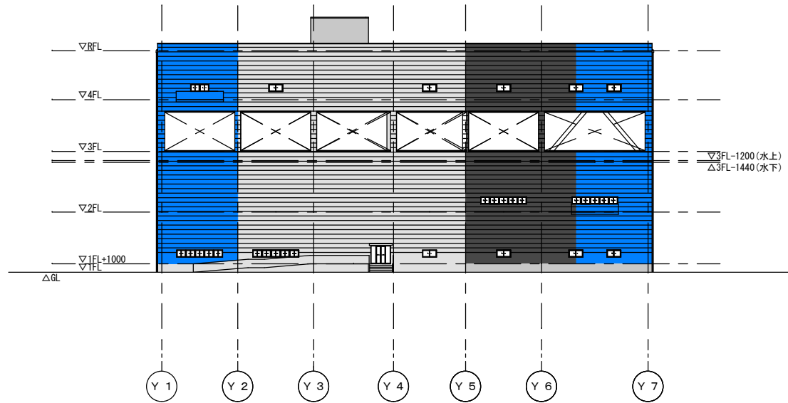
東側立面図
