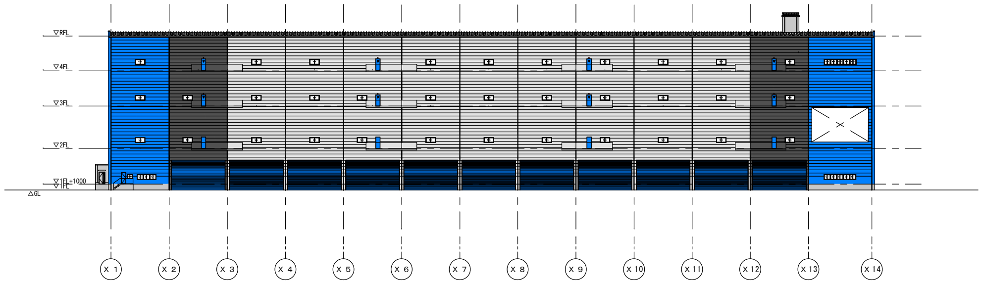
南側立面図
