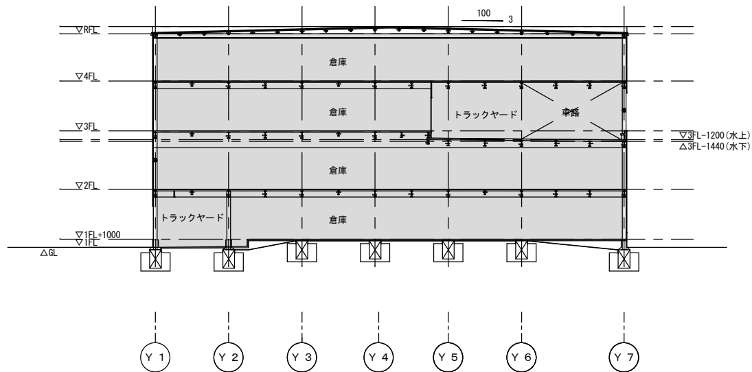
短辺断面図
